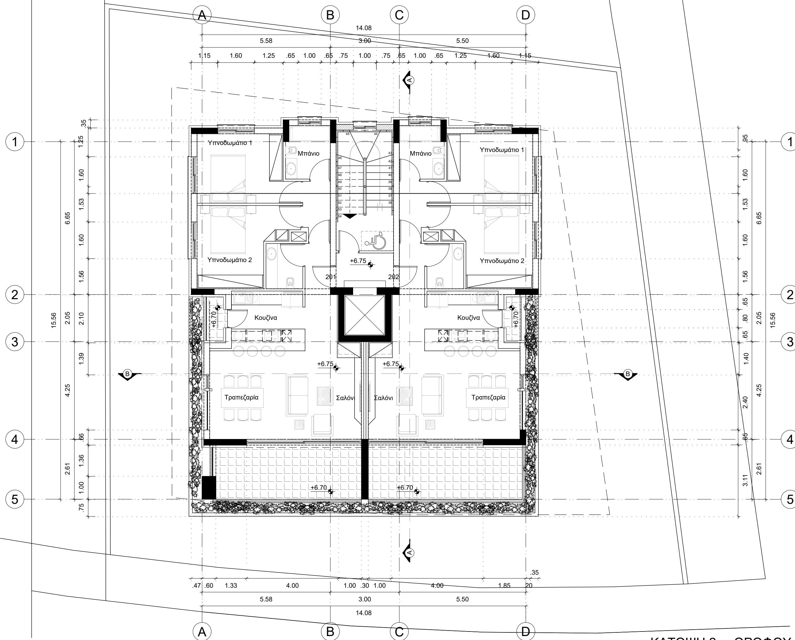
ΚΑΤΟΨΗ 2ου ΟΡΟΦΟΥ ΚΛ. 1:100
